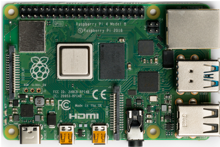
FIGURE 2 – Le Raspberry est un ordinateur basé sur un SoC. Le système sur puce est le carré argenté au centre.
