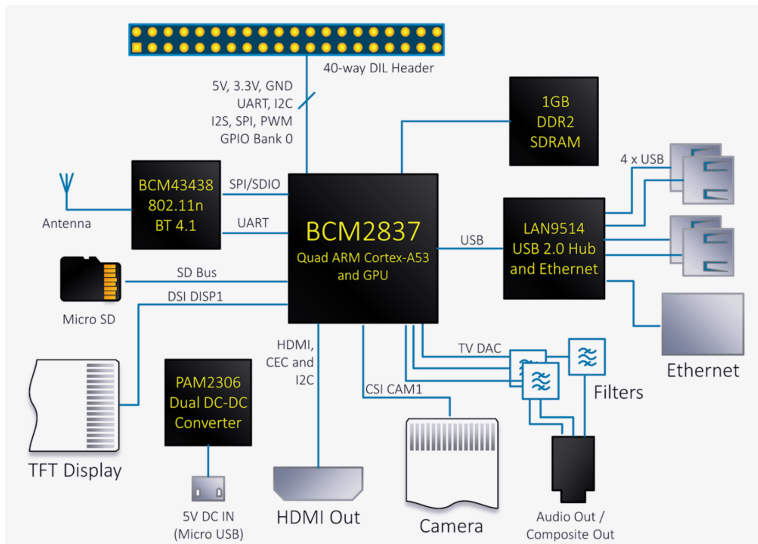
FIGURE 3 – Schéma du Raspberry
