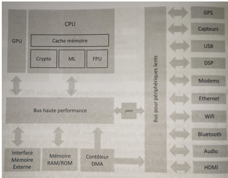
FIGURE 1 – Architecture d'un système sur puce
